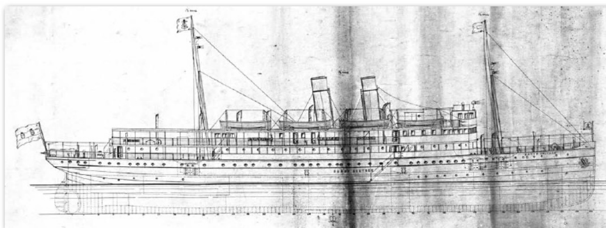
Nahoře: výrobni výlres loděnice Gourlay Brothers & Company v Dundeeve Skotsku v roce 1908. (sbírká Aloš Rlaš)
